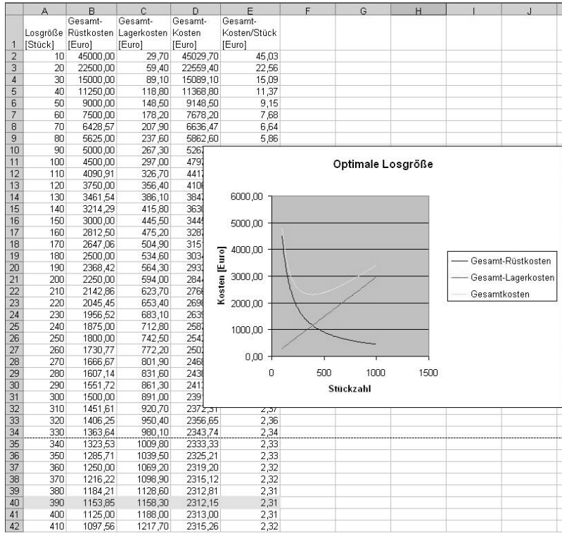
Bild 7-11 Testdatenauswertung
